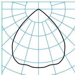
InperlaL G2 C07 HR22 1800-840 01 + RD-PC ■ C0 - C180 TX053064
