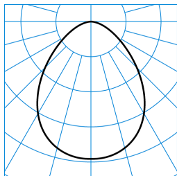
InperlaL G2 C07 HR22 1800-840 01 + DA-M 01 ■ C0 - C180 TX053063
