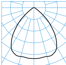
InperlaL G2 C07 HR22 1800-840 01 + ZN-PC ■ C0 - C180 TX053066
