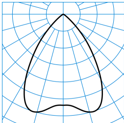
InperlaL G2 C07 HR19 1800-830 03 + DA 03 ■ C0 - C180 TX053008
