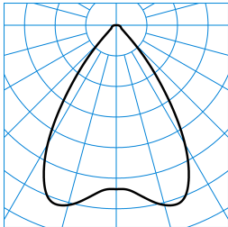
InperlaL G2 C07 HR19 1800-830 03 + ZN-PC ■ C0 - C180 TX053012
