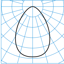
InperlaL G2 C07 HR19 1800-830 03 + DA-M 03 ■ C0 - C180 TX053009
