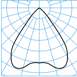
InperlaL G2 C07 HR19 1800-830 ETDD 03 ■ C0 - C180 TX769472
