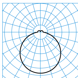
Olisq RWD2 DW 14-40/4/ML-830 ET IP54 PC (stage 3) TX842848
