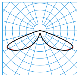
9821 RB6L-LR/3800-730 4G1S ET TX778559
