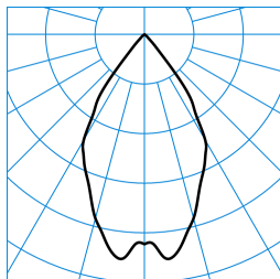
InperlaLP C05 BR19 1800-830 ETDD 01 ■ C0 - C180 TX771480
