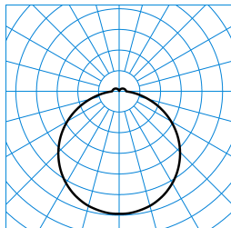
Olisq RWD3 DW 30-840 ET EB3 IP54 PC + Olisq RWD3 ZDR 1/2 01 TX426691
