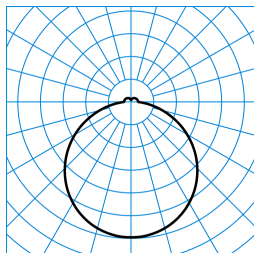
Olisq RWD3 DW 30-840 ET EB3 IP54 PC TX376134
