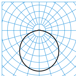
Olisq RWD3 DW 30-840 ET EB3 IP54 PC + Olisq RWD3 C 01 TX426451
