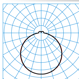
Olisq QWD2 DW 35-8TW ETDD8 (DWW) TX873186
