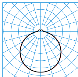
Olisq QWD2 DW 14-40/4/ML-840 IP54 ET (stage 2) TX776271
