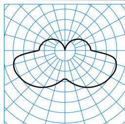
PolaronIQ WD2 LED3000-840 ET TX773690
