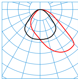
Cultega T COM PAW 600-9TW ETDI KL 01 (DWW) TX875497
