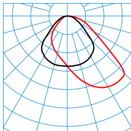
Cultega T COM PAW 600-9TW ETDI KL 01 (DSU) TX875482
