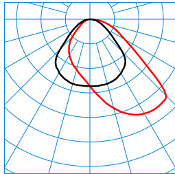
Cultega T COM PAW 600-9TW ETDI KL 01 (DCW) TX875489
