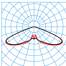
Publisca P2-RB6L-LRA/4600-740 6G1S ET (CLO initial value) TX300350
