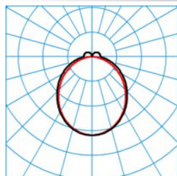
ELINE DSL120 840 L150 1 50
