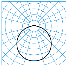
Olisq RWD2 DW 20-840 ETBLE +DMR IP54 PC + Olisq RWD2 ZDR 1/2 01 TX426069
