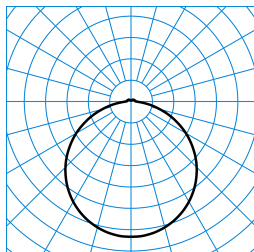
Olisq RWD4 DW 60-840 ETBLE +DMM IP54 + Olisq RWD4 ZDR 1/2 03 TX427501
