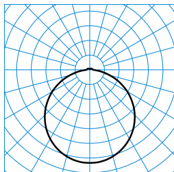
Olisq RWD4 DW 60-840 ETBLE +DMM IP54 + Olisq RWD4 ZDR 1/2 05 TX462814
