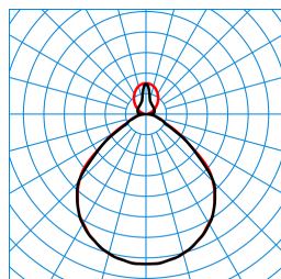
Luceos D/H2-L CDP 6500-840 ETDD 03 (Ceiling D2 ZD/03) TX877260
