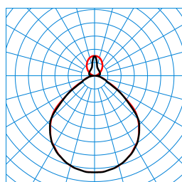
Luceos D/H2-L CDP 6500-840 ETDD 03 (Ceiling D2 ZD/03+EB3) TX277143
