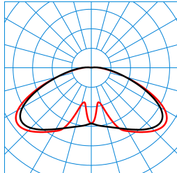
Publisca P1W-RBT-LR/1500-740 2G1S TX053568
