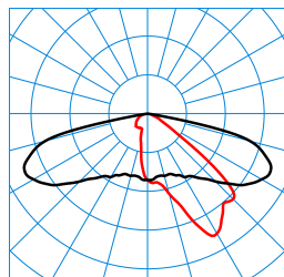
Cuvia 40-AB2L-LR/2600-740 4G1S ET TX778075
