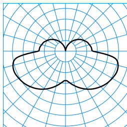
PolaronIQ WD2 LED3000-830 ETDD TX773683
