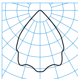
InperlaLP C05 HR22 1800-930 01 + ZN-PC ■ C0 - C180 TX045508
