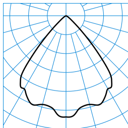
InperlaLP C05 HR22 1800-930 ETDD 01 TX768802
