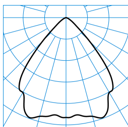
InperlaLP C05 HR22 1800-930 01 + RD-PC TX045506
