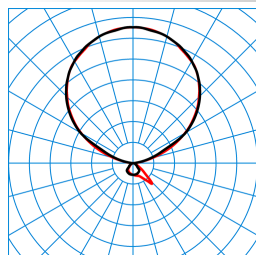
Luceos S-T PAW-IL 300-840 ETDD 05 (LEO1) TX877126
