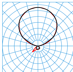
Luceos S-T PAW-IL 300-840 ETDD 05 (LEO2) TX877111
