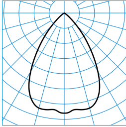
InperiaL G2 C07 BR22 3800-840 ETDD 03 ■ C0 - C180 TX769025
