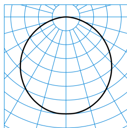
Olisq RWD4 DW 60-840 ETDD PC + Olisq RWD4 ZDR 1/1 01 TX427226
