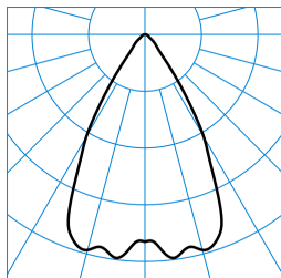
InperlaLP C05 HR19 1800-930 01 + RG-PC ■ C0 - C180 TX045499
