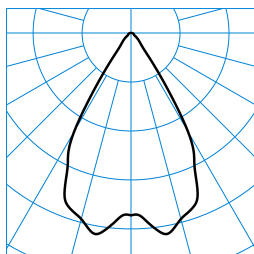
InperlaLP C05 HR19 1800-930 01 + ZN-PC ■ C0 - C180 TX045500
