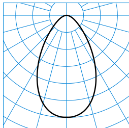
InperlaLP C05 HR19 1800-930 01 + DA-M 01 ■ C0 - C180 TX045496
