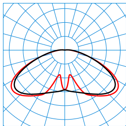
Publisca P1W-RBT-LR/1800-730 2G1S ET (CLO initial value) TX301776
