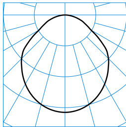
Onplana D11 OTA25 4000-8TW ETDD8 26 (DWW) TX874450
