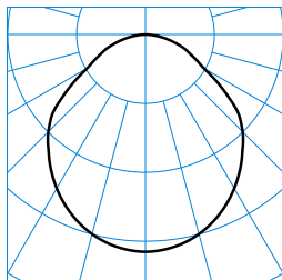
Onplana D11 OTA25 4000-8TW ETDD8 26 (DSU) TX874449
