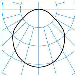
Onplana D11 OTA25 4000-8TW ETDD8 26 (DCW) TX874448
