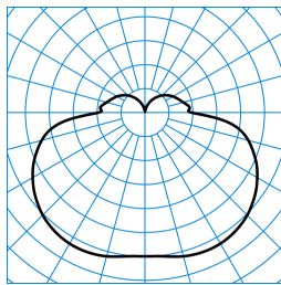
PolaronIQ WD2D LED3000-840 ETDD TX773763
