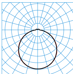
Olisq QWD3 DW 45-830 ETDD IP54 + Olisq QWD3 ZDR 1/2 03 TX461283
