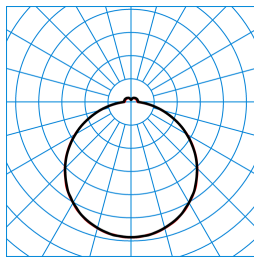
Olisq QWD3 DW 45-830 ETDD IP54 TX376265
