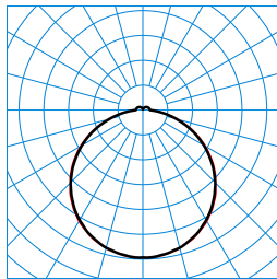
Olisq QWD3 DW 45-830 ETDD IP54 + Olisq QWD3 ZDR 1/2 01 TX462040
