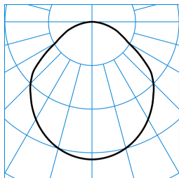
Onplana D09 OTA25 3000-8TW ETDD8 01 (DCW) TX874433
