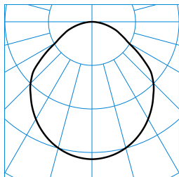
Onplana D09 OTA25 3000-8TW ETDD8 01 (DSU) TX874434
