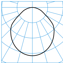
Onplana D09 OTA25 3000-8TW ETDD8 01 (DWW) TX874435
