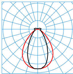
TugraHE+ 12 PN 80-830 ET PC C2 TX558367
