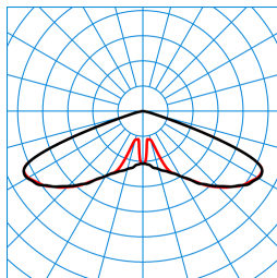
Publisca P1-RB6L-LRA/1650-730 2G1S ET (CLO end value) TX301491
