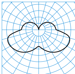
PolaroniQ WD1 LED1000-830 ETDD TX773535
