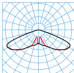
Publisca P1-RB6L-LR/1200-730 2G1S ET (CLO end value) TX301862
