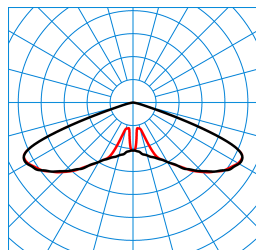
Publisca P1-RB6L-LR/1200-730 2G1S TX047618
