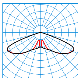
Publisca P1-RB6L-LR/1200-730 2G1S ET (CLO initial value) TX301772
