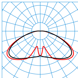
Publisca P1W-RBT-LR/1800-740 2G1S ET (CLO end value) TX300295
