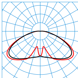
Publisca P1W-RBT-LR/1800-740 2G1S ET (CLO initial value) TX300202
