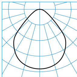
Onplana D11 CDP19 4000-830 ETDD 01 TX771996
