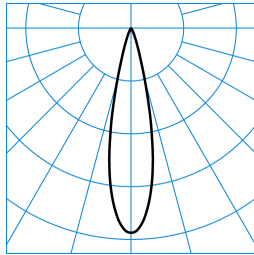
7651 Lentyp L-SP 40-830 M33 ETBLE 05 (150) TX782517
