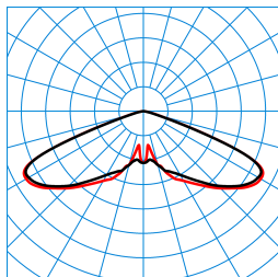
Publisca P2-RB6L-LR/3800-740 6G1S ET (CLO initial value) TX300194
