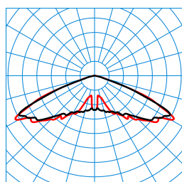
Publisca P1W-RB6L-LR/1500-740 2G1S ET (CLO initial value) TX301424
