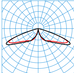
CS 19 100-RB6L-LR/1200-740 2G1S ET (CLO end value) TX300069
