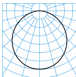
Olisq RWD2 DW 20-830 ET + Olisq RWD2 ZDR 1/1 01 TX425883
