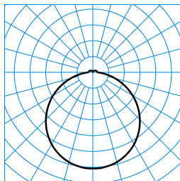
Olisq RWD2 DW 20-830 ET + Olisq RWD2 ZDR 1/2 03 TX427721
