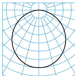
Olisq RWD4 DW 40-830 ETBLE +DMR IP54 + Olisq RWD4 ZDR 1/1 01 TX427148
