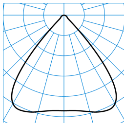
Mirona Fit R LW 350-865 ET SLR3 TX843221
