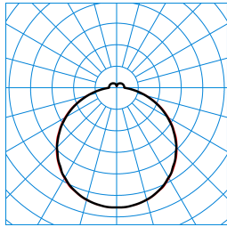
Olisq QWD2 DW 14-40/4/ML-840 ET IP54 IK (stage 0) TX842846
