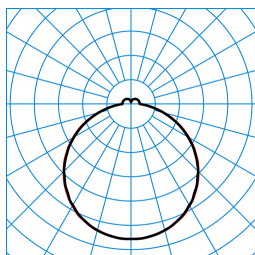
Olisq QWD2 DW 14-40/4/ML-840 ET IP54 IK (stage 3) TX842844
