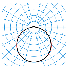
Olisq QWD2 DW 14-40/4/ML-840 ET IP54 IK + Olisq QWD2 ZDR 1/2 01 (stage 0) TX843020
