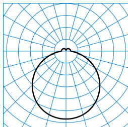
Olisq RWD2 DW 20-840 ET EB3 TX375797
