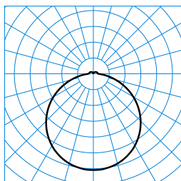
Olisq RWD2 DW 20-840 ET EB3 + Olisq RWD2 ZDR 1/2 05 TX429207
