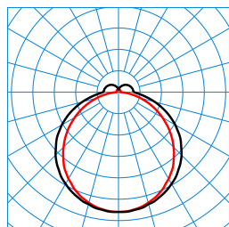
Olisq LWD3 DW 75-8TW ETDD8 (DSU) TX873082
