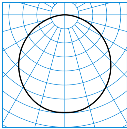
Olisq RWD1 DW 20-840 ETDD IP54 PC + Olisq RWD1 ZDR 1/1 01 TX425657
