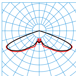
Publisca P1-RB6L-LRA/3200-730 4G1S ET (CLO initial value) TX300184
