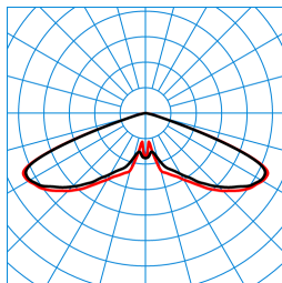
Publisca P1-RB6L-LRA/3200-730 4G1S ET (CLO end value) TX300887
