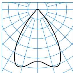
InperiaL G2 C07 HR19 1000-830 03 + ZN-PC ■ C0 - C180 TX052988
