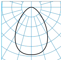
InperiaL G2 C07 HR19 1000-830 03 + DA-M 03 ■ C0 - C180 TX052985
