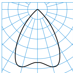
InperiaL G2 C07 HR19 1000-830 03 + RD-PC ■ C0 - C180 TX052986
