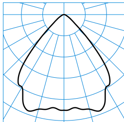
InperiaLP C05 HR22 1800-940 01 + RG-PC TX045509
