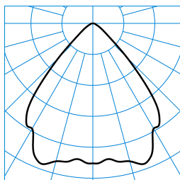
InperiaLP C05 HR22 1800-940 01 + DA 03 TX045489
