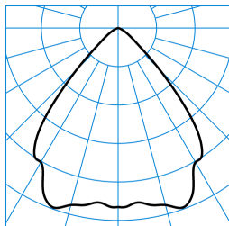
InperiaLP C05 HR22 1800-940 01 + RD-PC TX045492
