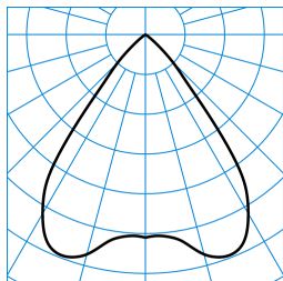
InperlaL G2 C07 HR19 2700-830 ETDD 03 ■ C0 - C180 TX769672
