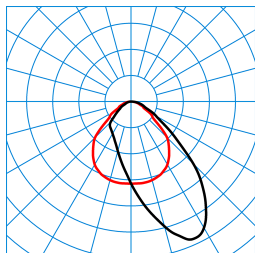
Luceos D/H2-L CDP-A 5000-840 ETDD 03 (Ceiling D2 ZD/03+EB3) TX277138
