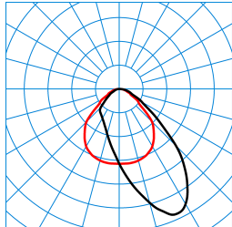
Luceos D/H2-L CDP-A 5000-840 ETDD 03 (Ceiling D2 ZD/03) TX877262
