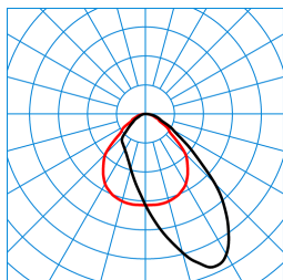
Luceos D/H2-L CDP-A 5000-840 ETDD 03 (Pendant ZS/ZST+EB3) TX245968
